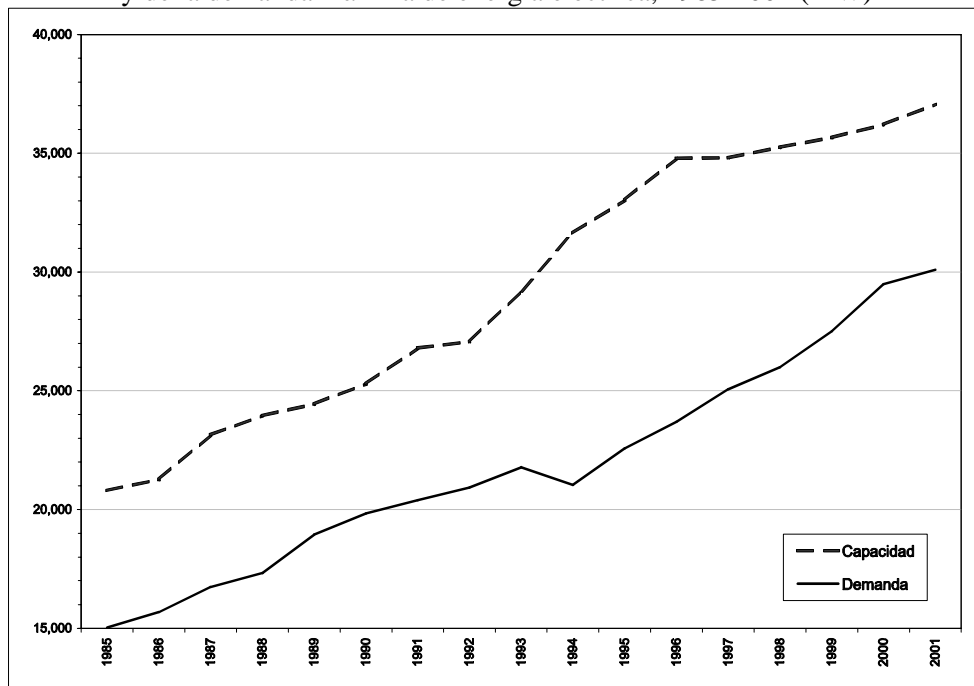
Figura 1: Evolución de la capacidad efectiva de generación y de la demanda máxima de energía eléctrica, 1985-2001 (MW)
