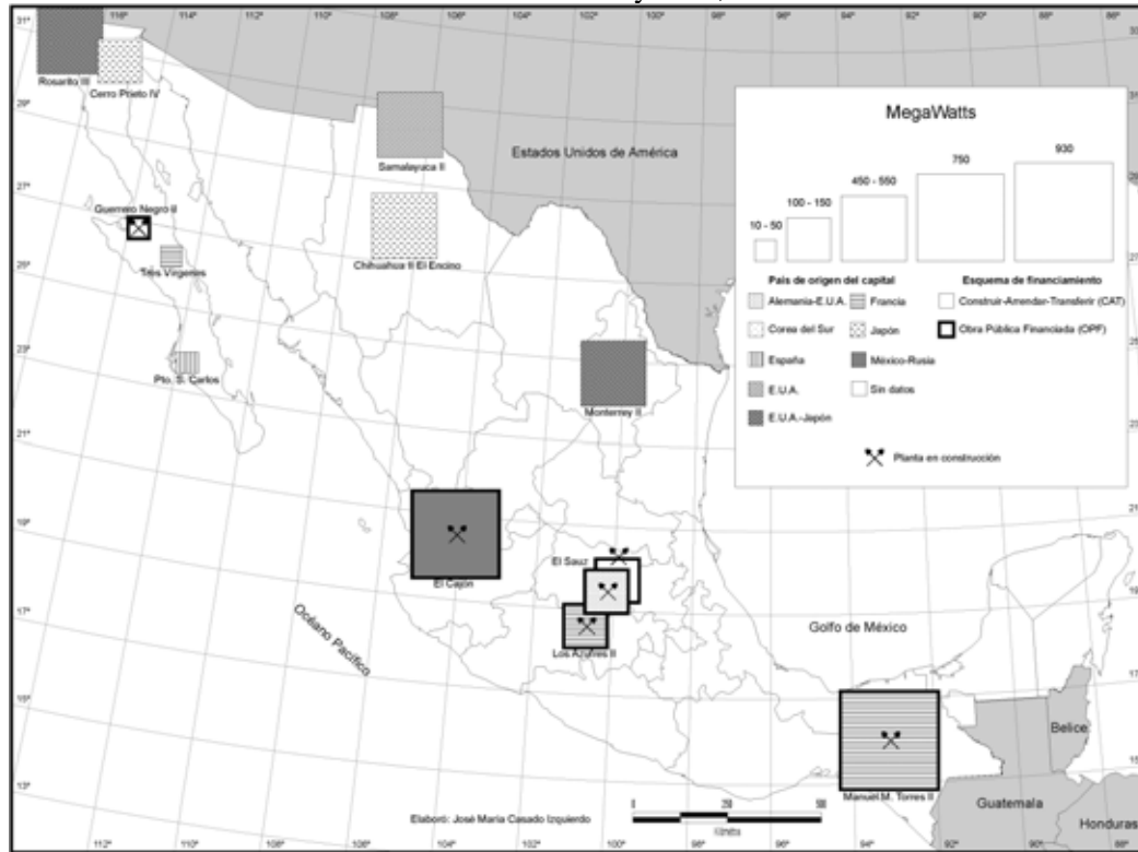
Figura 10. Centrales eléctricas promovidas por CFE con inversión privada mediante los esquemas de financiamiento CAT y OPF, 2002
